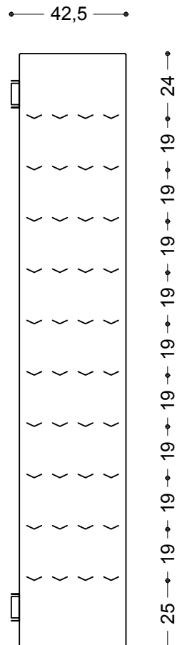
SEZIONE LATERALE
