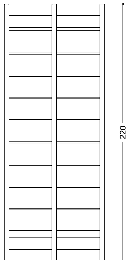
PROSPETTO FRONTALE
