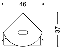
VISTA DALL'ALTO
